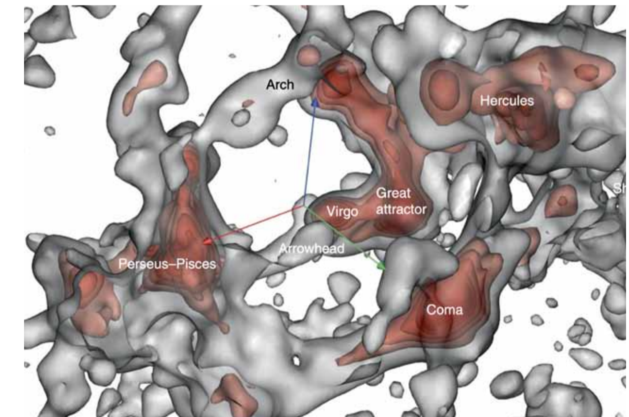
Welt der Galaxien im kosmischen Netzwerk der dunklen Materie
